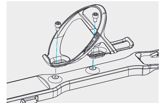
zu 1. Flaschenhalter befestigen
