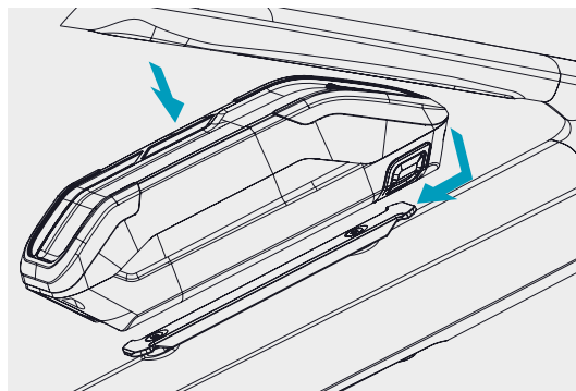
zu 2. Auf die Dockingschiene setzen und gleichzeitig nach unten schieben
