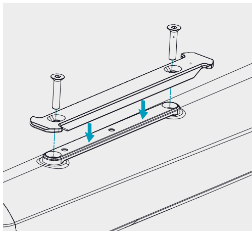
zu 1. Dockingschiene montieren
