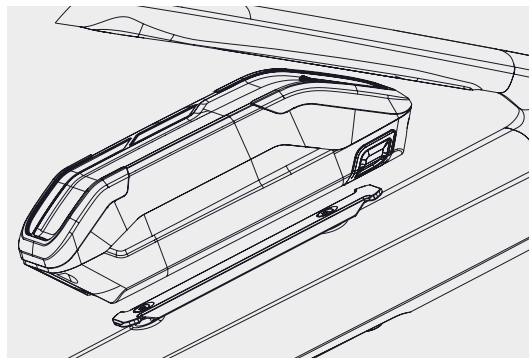
zu 1. An die Dockingschiene halten
